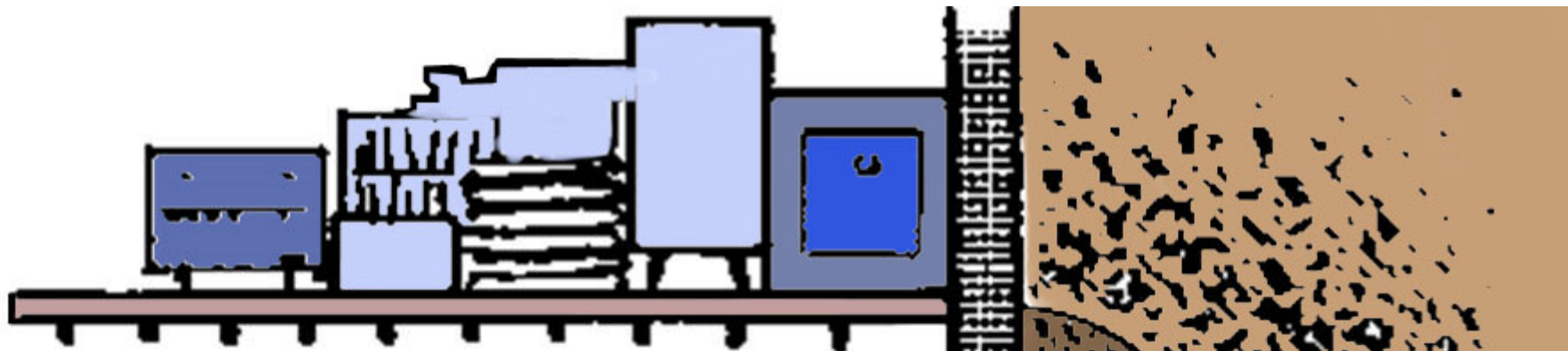
Устройство противорадиационного укрытия в полуподвальном помещении
